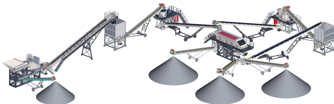
Модульный комплекс 3-этапной обработки System 200 (щековая дробилка – конусная дробилка – грохот – ударная дробилка с вертикальным валом)
