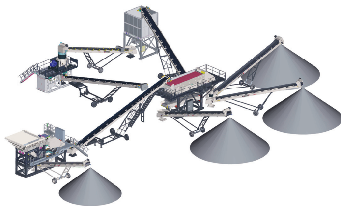
Модульный комплекс 2-этапной обработки System 200 (щековая дробилка – грохот – конусная дробилка)
