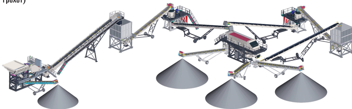
Модульный комплекс 3-этапной обработки System 200 (щековая дробилка – конусная дробилка – грохот – конусная дробилка)
