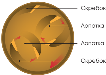
Модели RP1000 - RP1500 – две смесительные звездочки
