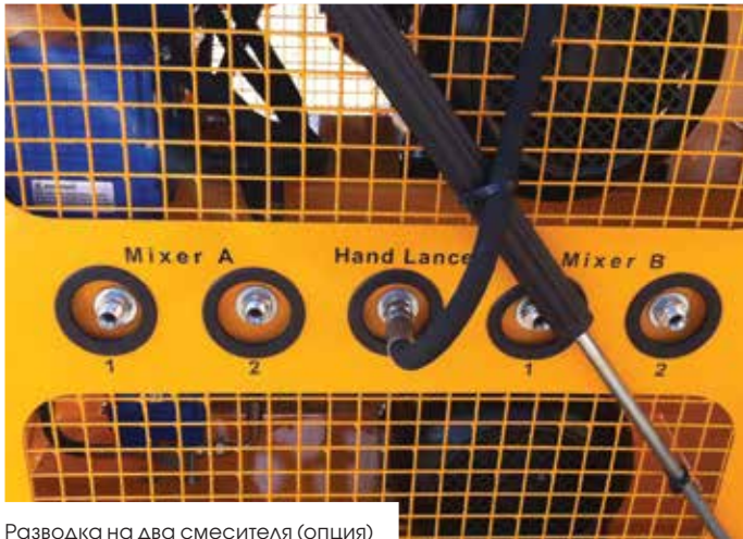
Разводка на два смесителя (опция)
