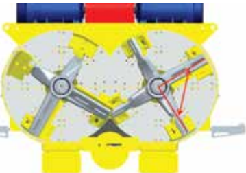
Крепление рукоятей под углом 90°
