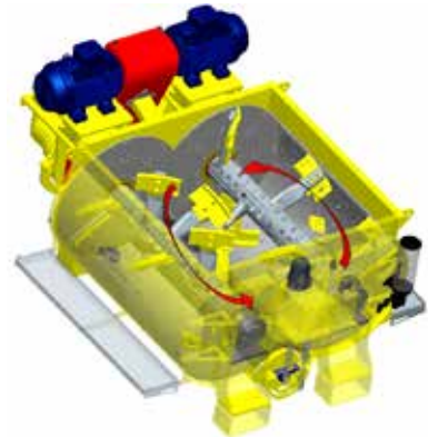
Движение материала в смесителе
