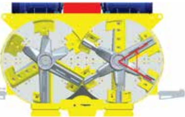
Крепление рукоятей под углом 60°
