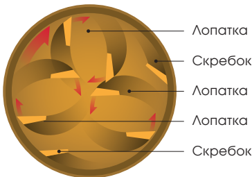
Модели RP2000 - RP3000 – три смесительные звездочки
